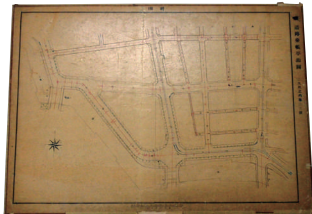
道路基帳平面図（神田）
